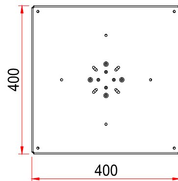
PIANTA scala 1:10
