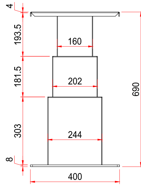
PROSPETTO APERTO scala 1:10
